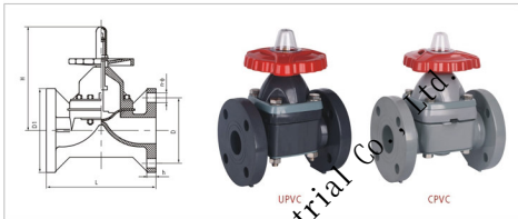
外形尺寸表 Dimension List
