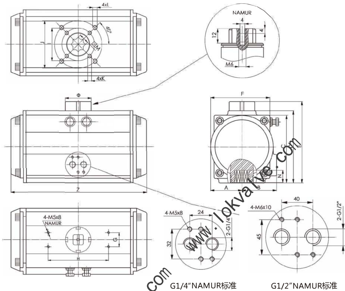
执行器安装尺寸表
