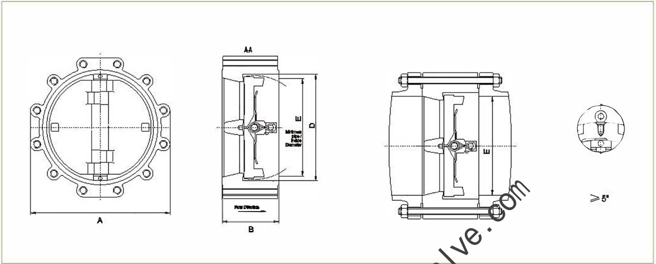
Lug type
